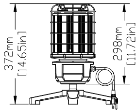
3. Floor stand
